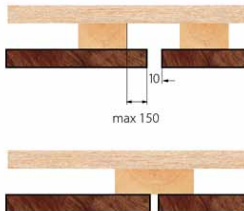
Figuur 9: Bevestiging
