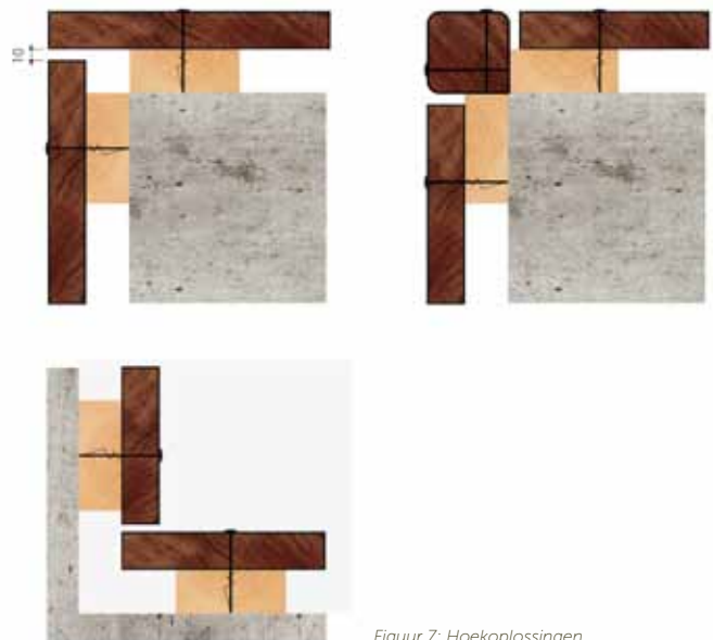
Figuur 7: Hoekoplossingen
